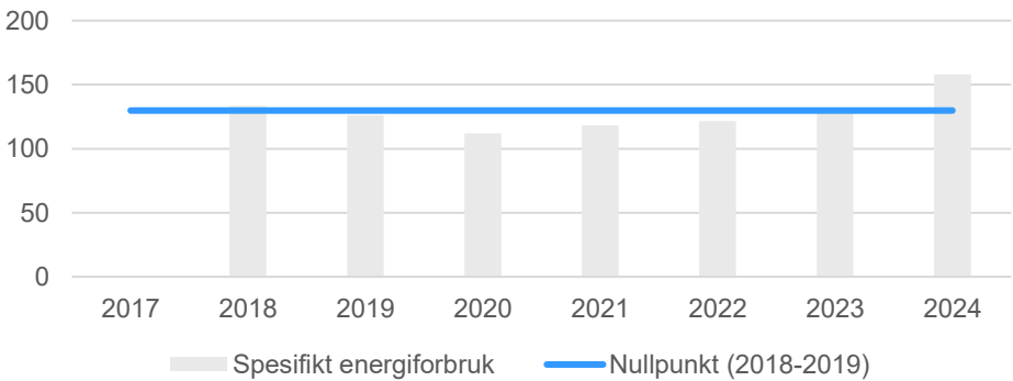
Utvikling spesifikk energiforbruk [kWh/m²]
